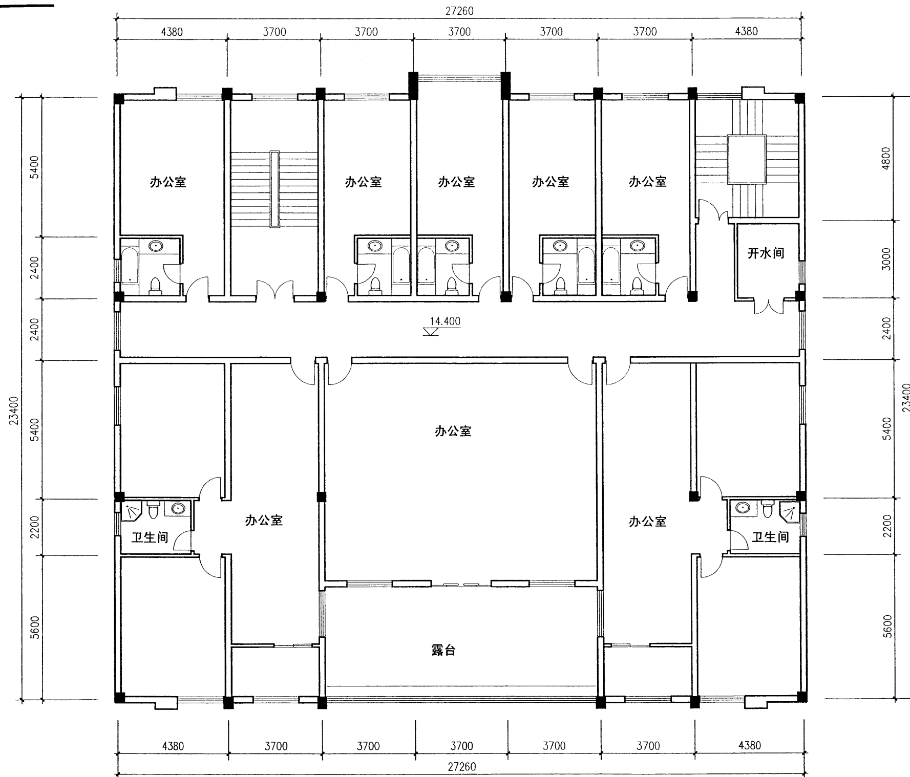
五层平面图
