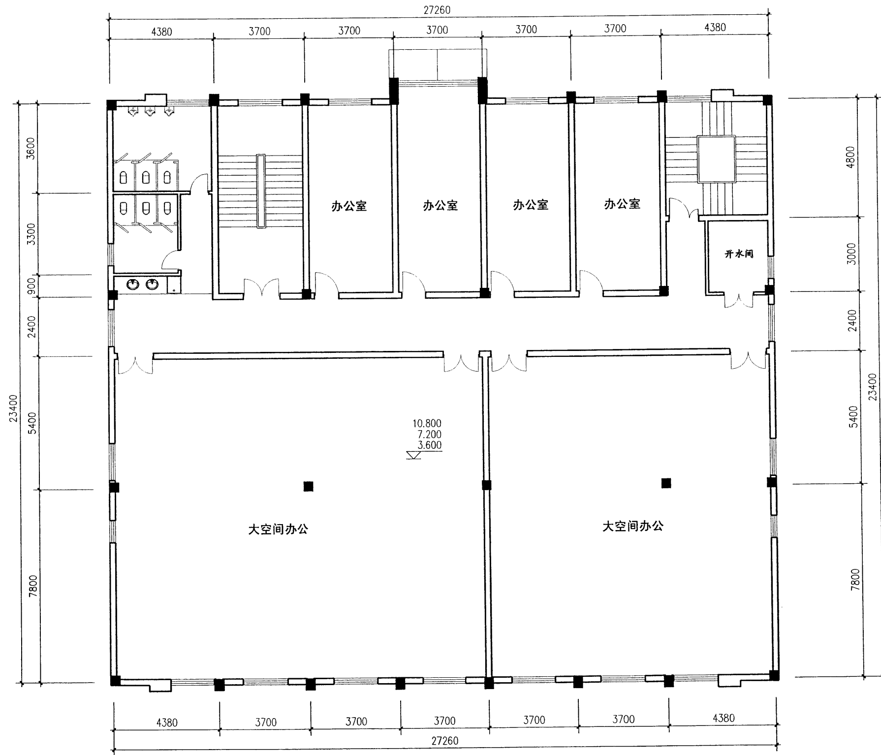
二~四层平面图
