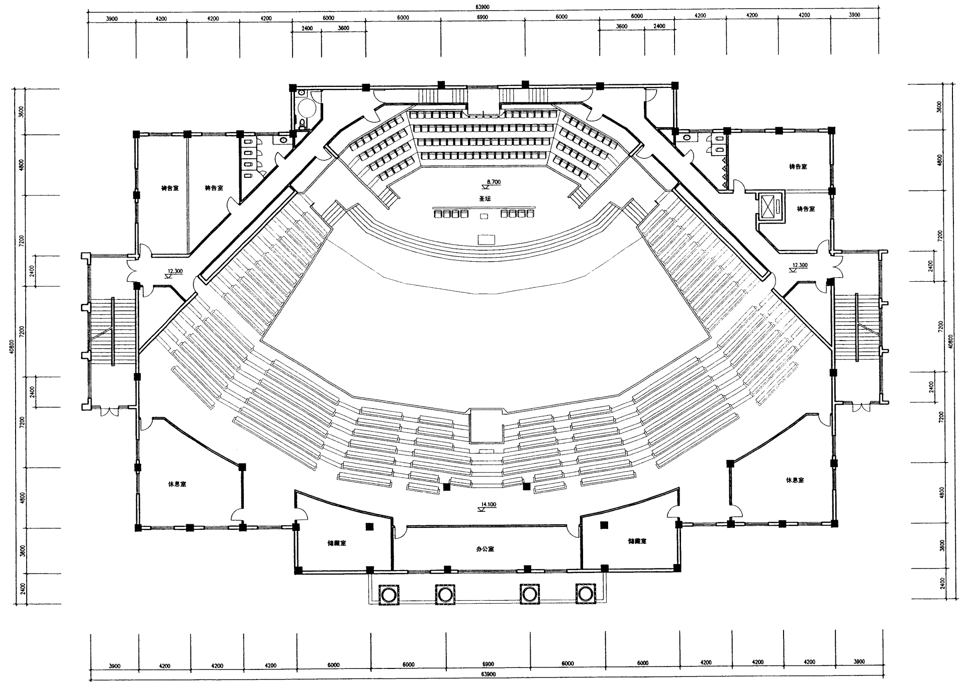
三层平面图
