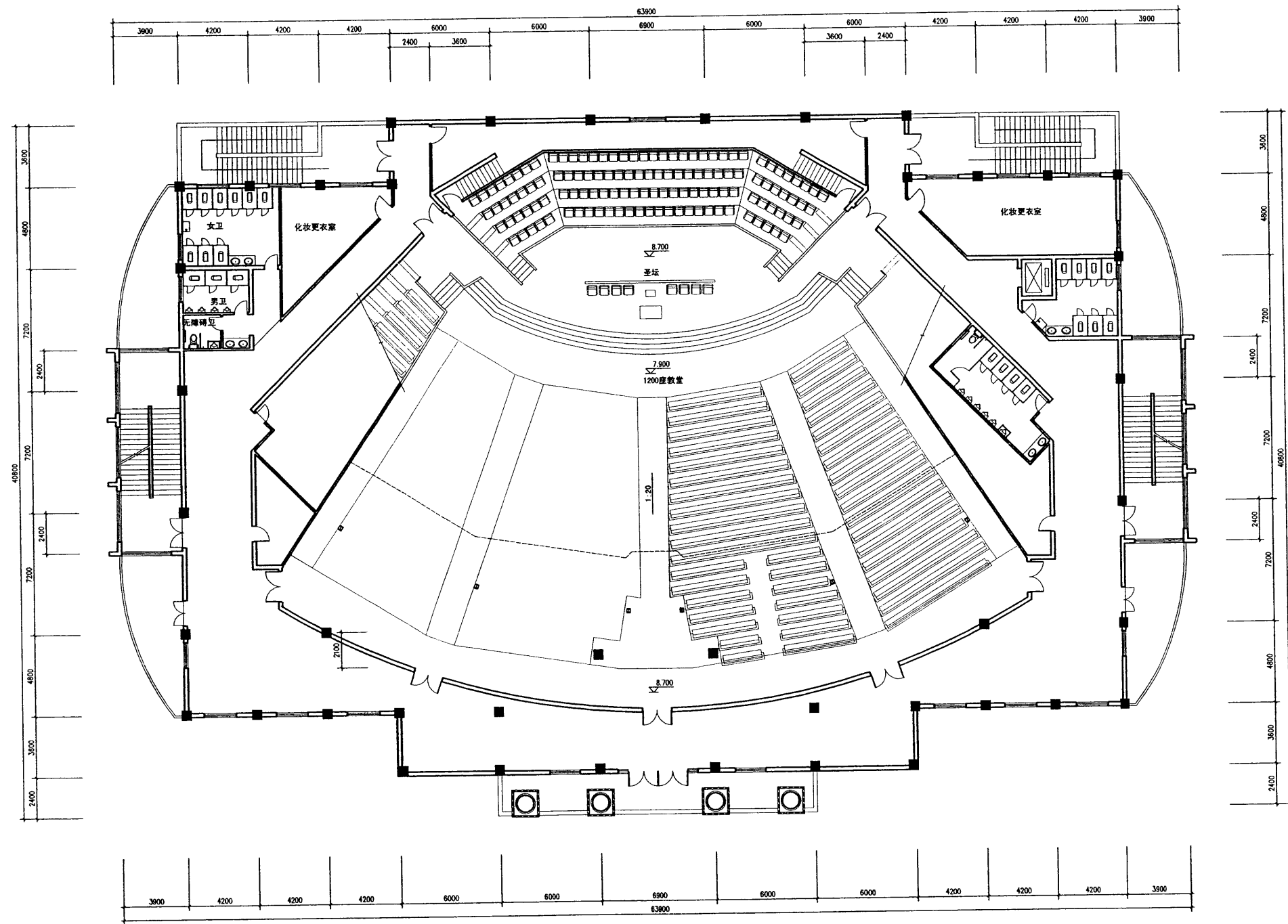
二层平面图
