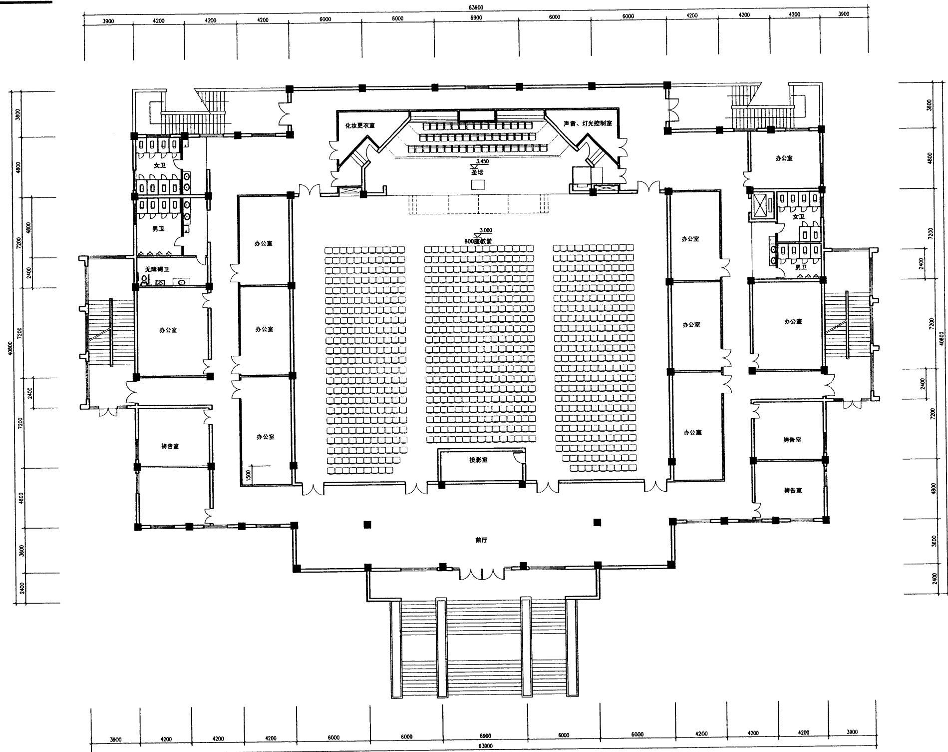
一层平面图
