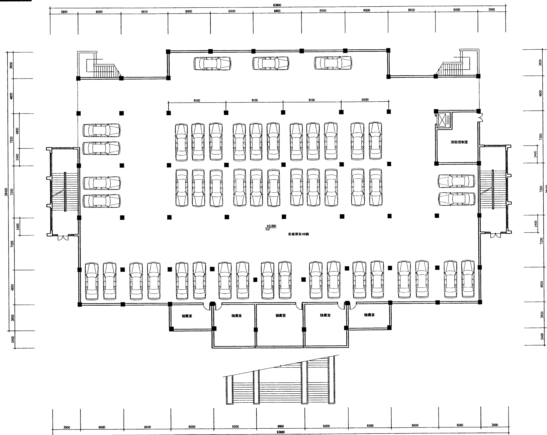
架空层平面图
